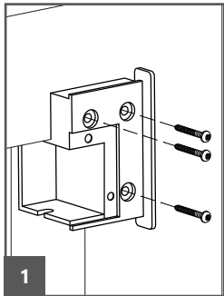
Sido beslag | Side brackets
